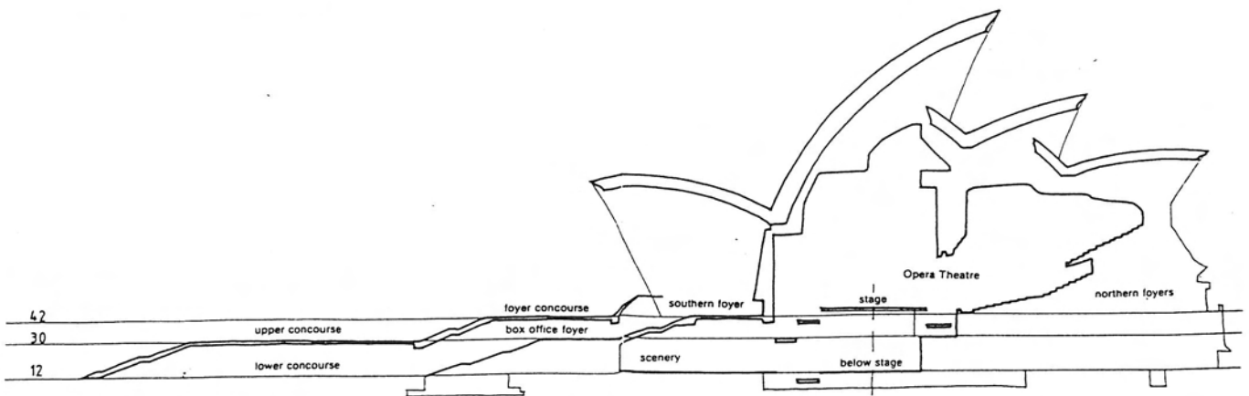
Thiết đồ xuyên Opera Theatre (Hình 4)
